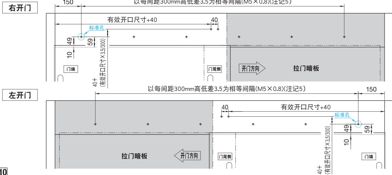
螺孔加工图(从检查口视图)
